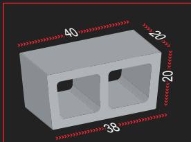
Hourdy 40x20x20x38 cm
