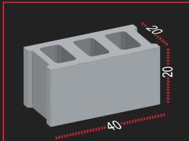
Hollow 20x20x40 cm
