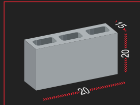
Hollow 15x20x20 cm
